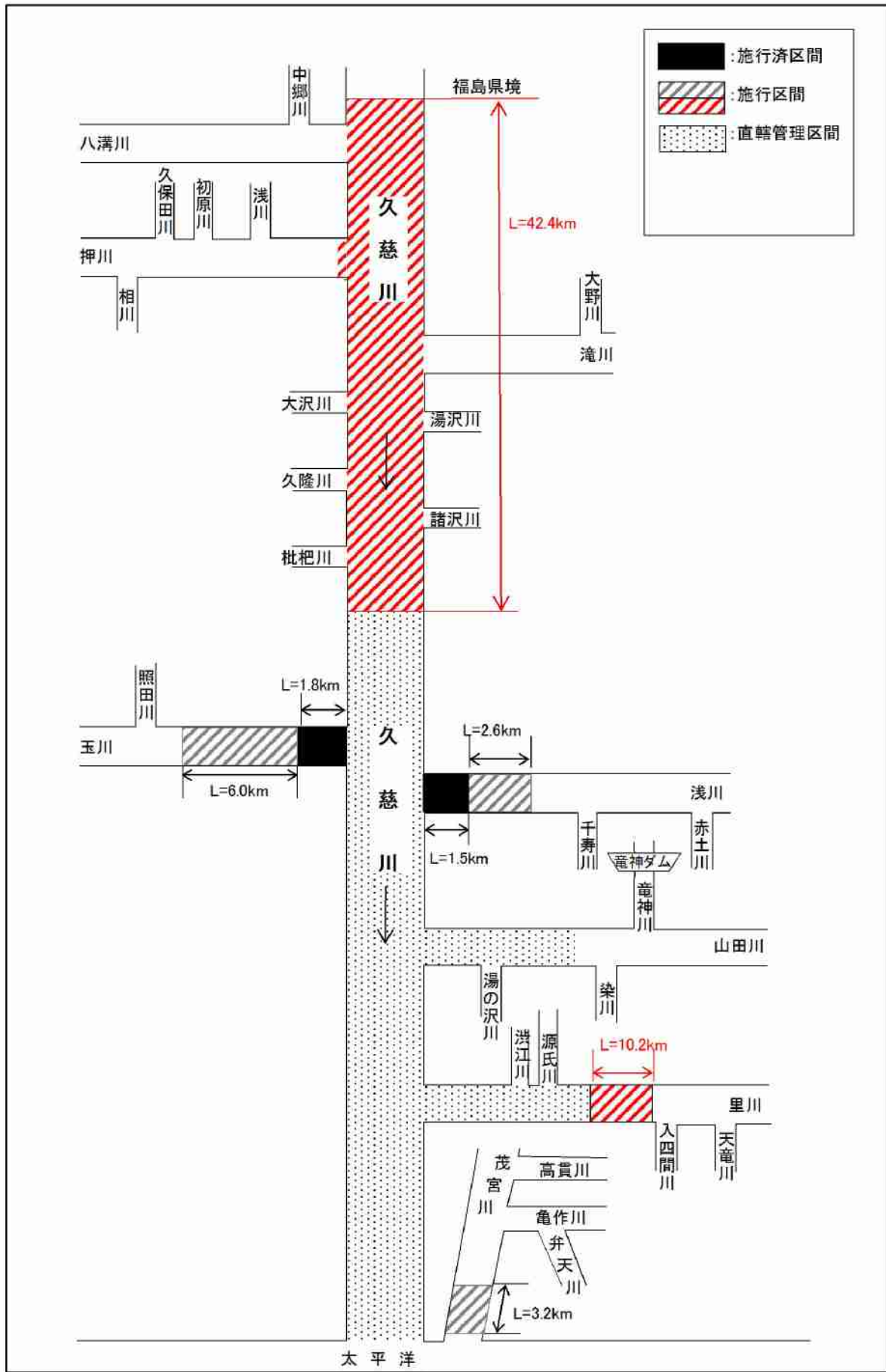
図-2.2 河川工事の施行区間模式図
