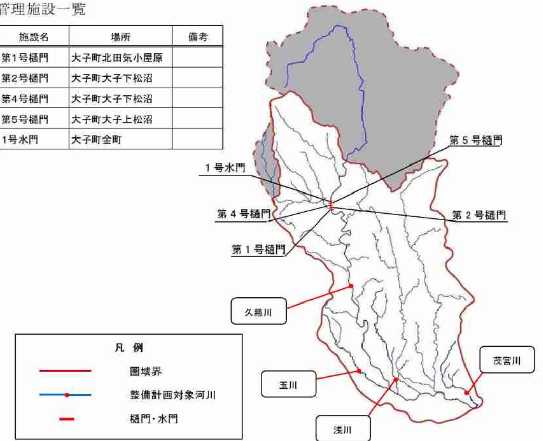
図-2.5 主な河川管理施設の位置図
