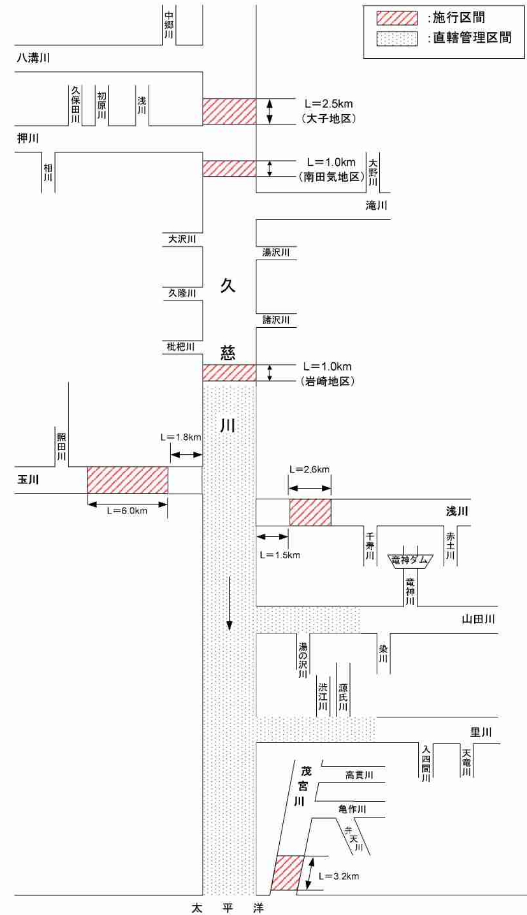
図-2.2 河川工事の施行区間模式図
