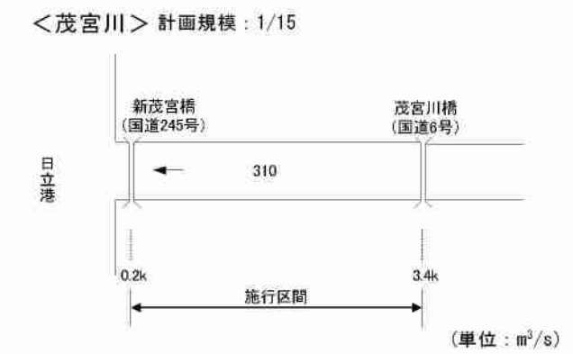
図-2.3 各河川の流量配分図及び代表断面図
