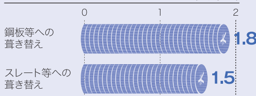
軽い屋根材への葺き替え
