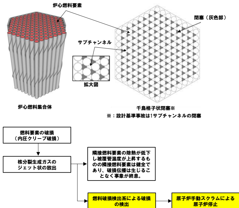
炉心損傷防止対策の概念図
