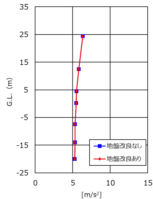
Ss-D(UD方向)
