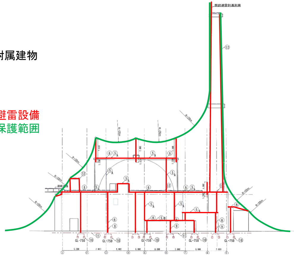
原子炉建物(格納容器を含む。)及び原子炉附属建物
