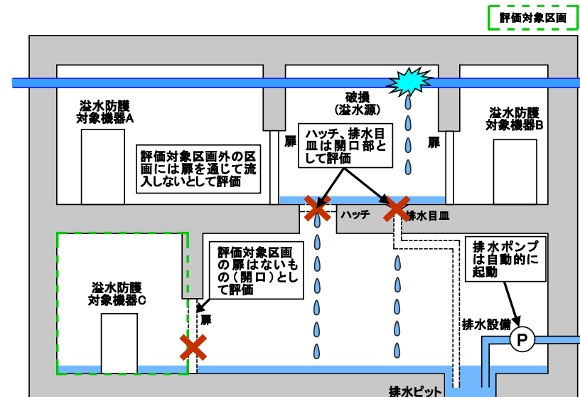
溢水評価の概要イメージ
