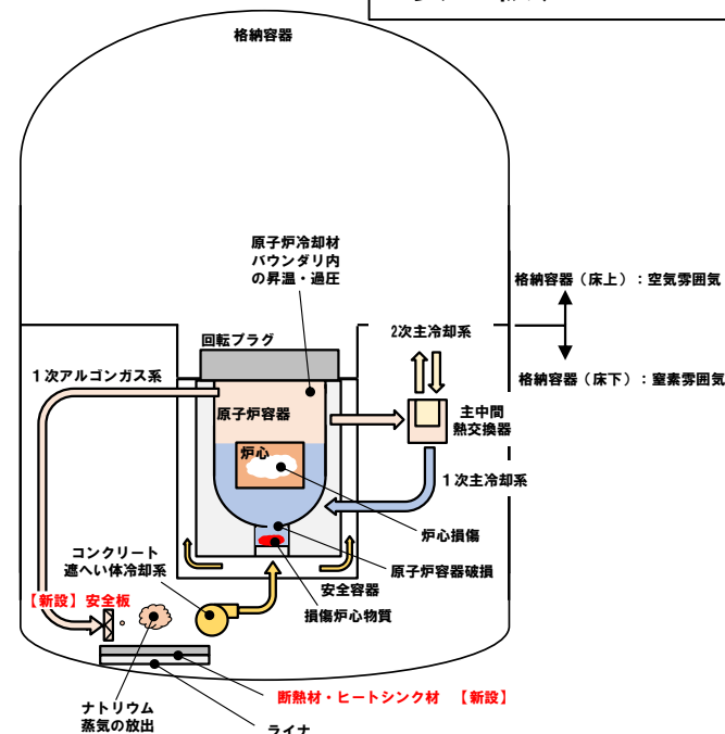
格納容器破損防止対策の概念図
