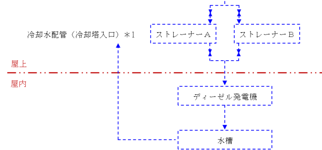
非常用ディーゼル電源系の冷却塔における降下火砕物流入防止板等の設置イメージ
