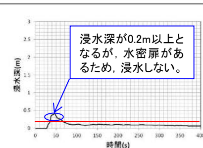
①原子炉建屋 (機器搬入口前)
