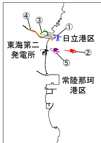
基準津波 (防波堤なし) ①～⑤の軌跡
