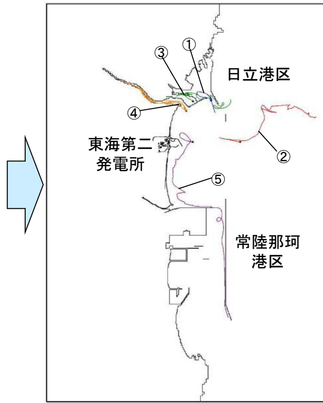
①～⑤の軌跡(防波堤あり)
