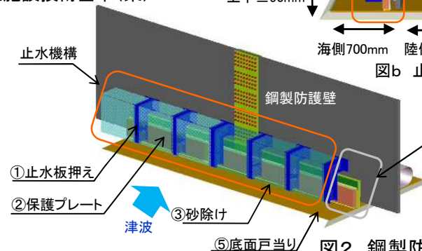
図a 止水機構の構造
