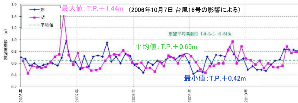
各月の朔望平均潮位の水位(満潮位)
