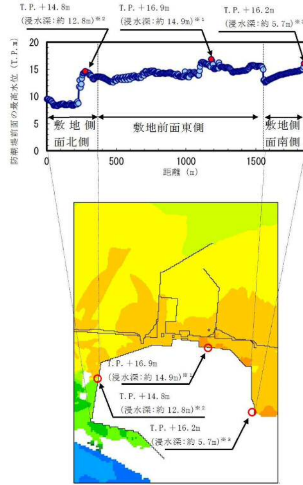
②「地盤沈下あり」, 「防波堤あり」のケース
