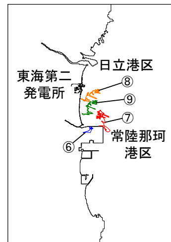
基準津波 (防波堤なし) ⑥～⑨の軌跡
