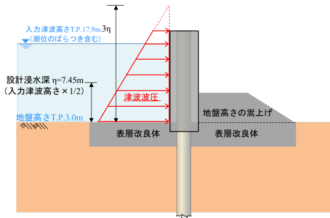
津波荷重の作用イメージ図(入力津波 × 1/2) 津波対策-157
