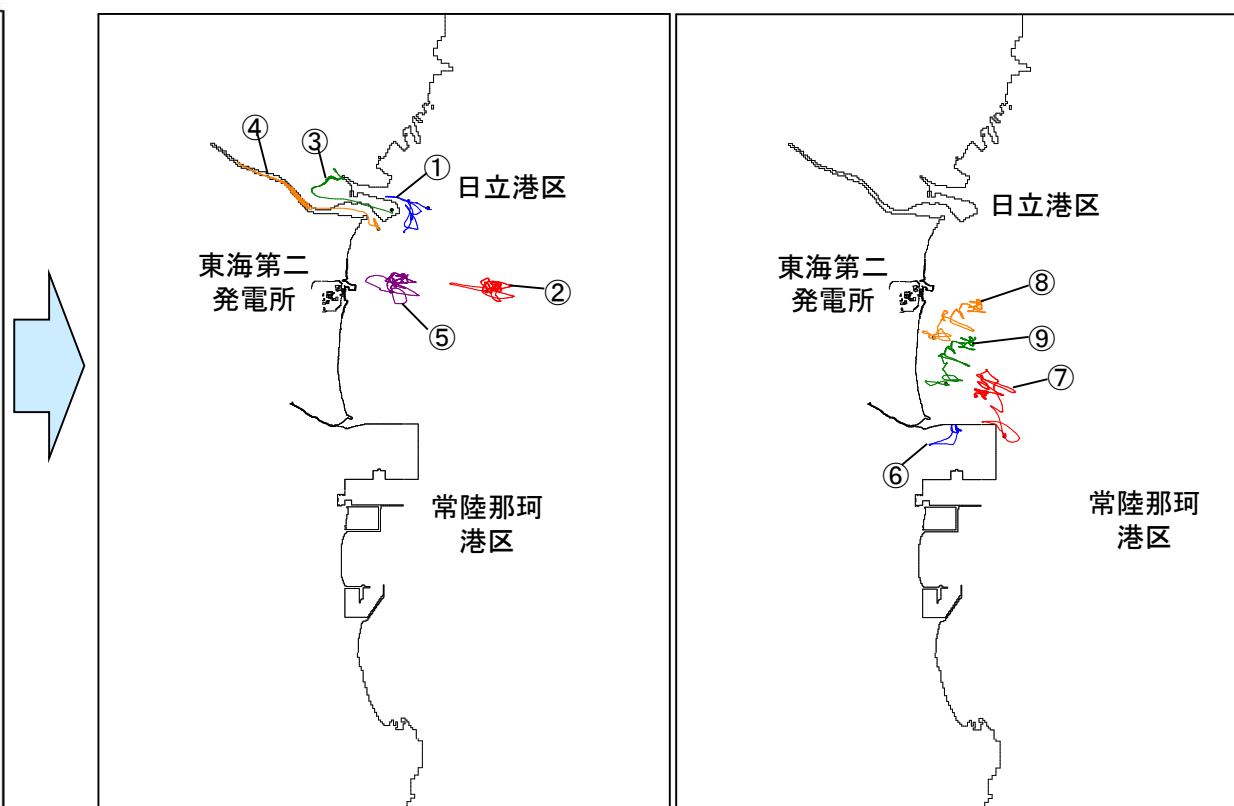
①～⑤の軌跡(防波堤なし)
