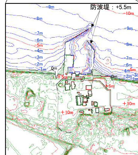
港湾部の防波堤効果有り
