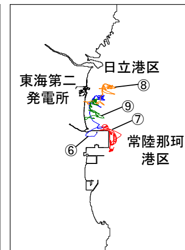
敷地に遡上する津波 (防波堤なし) ⑥～⑨の軌跡
