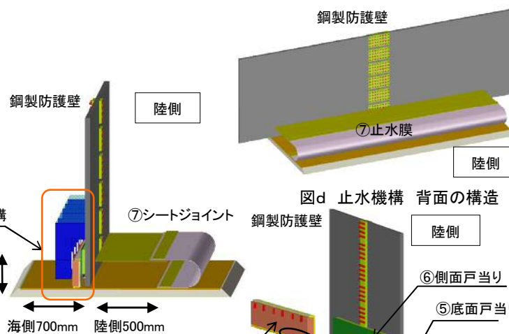
図b 止水機構断面図
