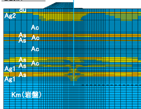
過剰間隙水圧比カウンター図
