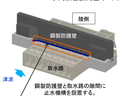
図1 鋼製防潮壁の構造
