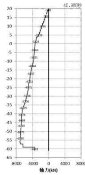
軸力 (kN)
