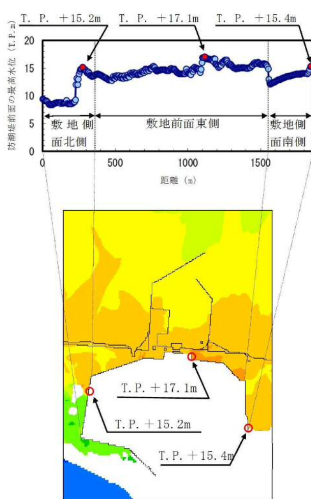
①「地盤沈下なし」, 「防波堤あり」のケース
