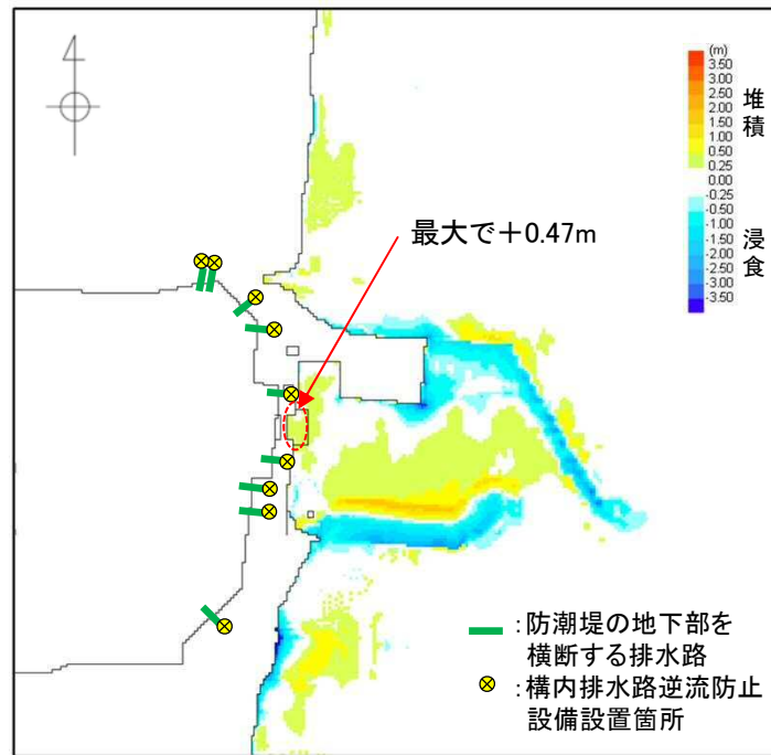
基準津波による砂の堆積・浸食分布と構内排水路逆流防止設備の位置 津波対策-171
