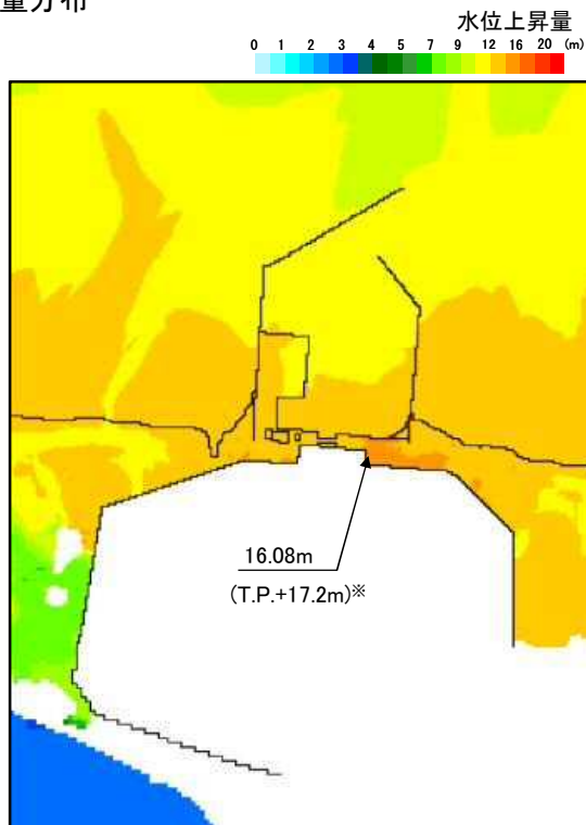
防潮堤設置ルート変更前
