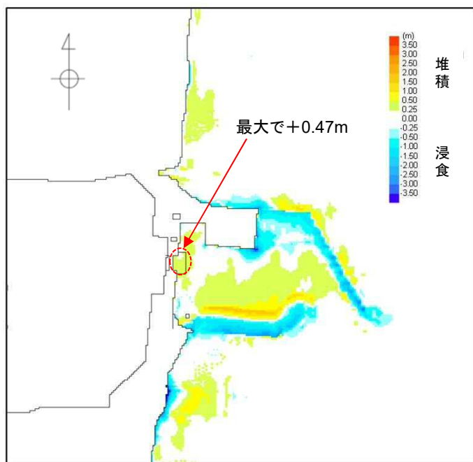
基準津波による砂の堆積・浸食分布
