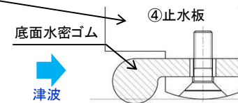
図e 底面水密ゴムの構造(断面図) 側面も同様に水密ゴムを設置
