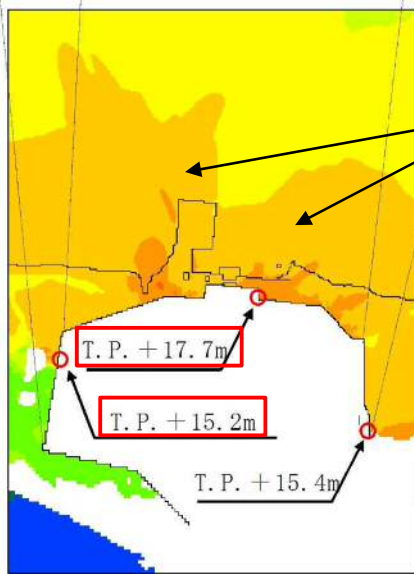
③「地盤沈下なし」, 「防波堤なし」のケース
