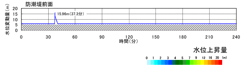
港湾部の防波堤効果有り
