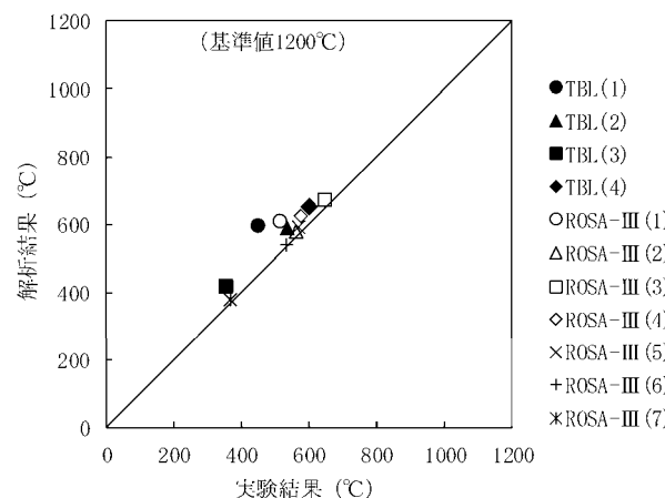
燃料被覆管最高温度
