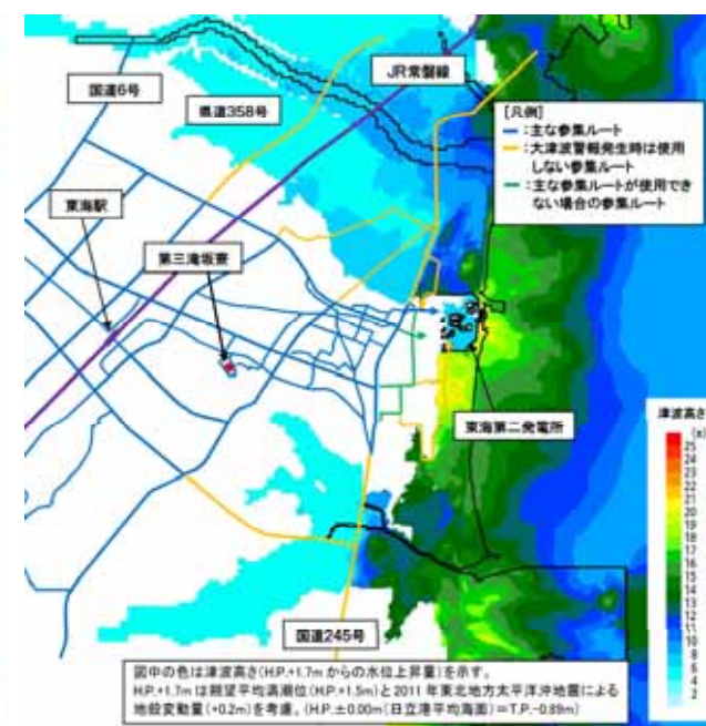
敷地に遡上する津波の遡上範囲想定図
