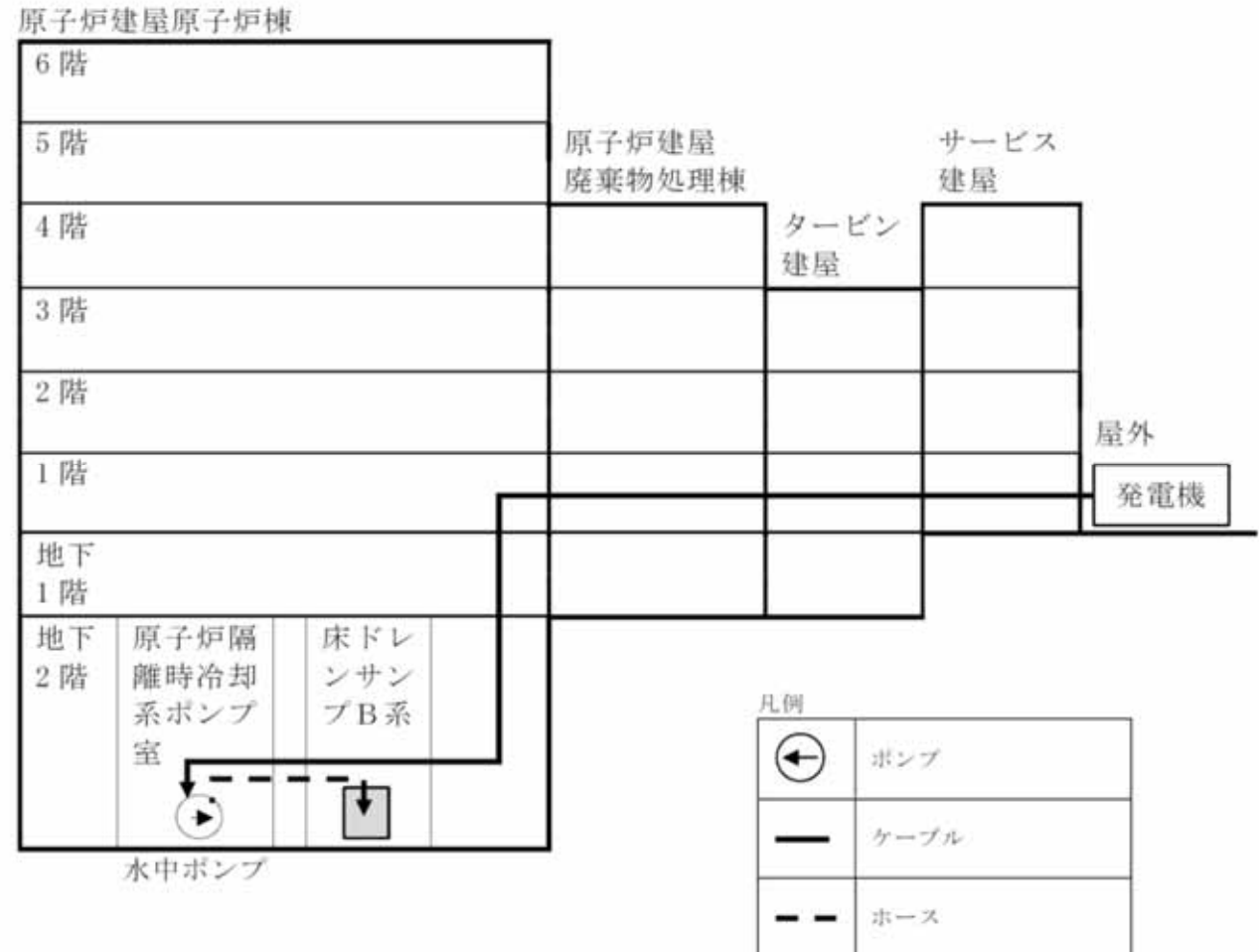
現場手動操作による原子炉隔離時冷却系の起動(排水処理) 概要図
