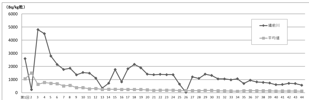
放射性セシウム (セシウム 134+セシウム 137) 濃度が最も高かった備前川の測定値と平均値の推移
