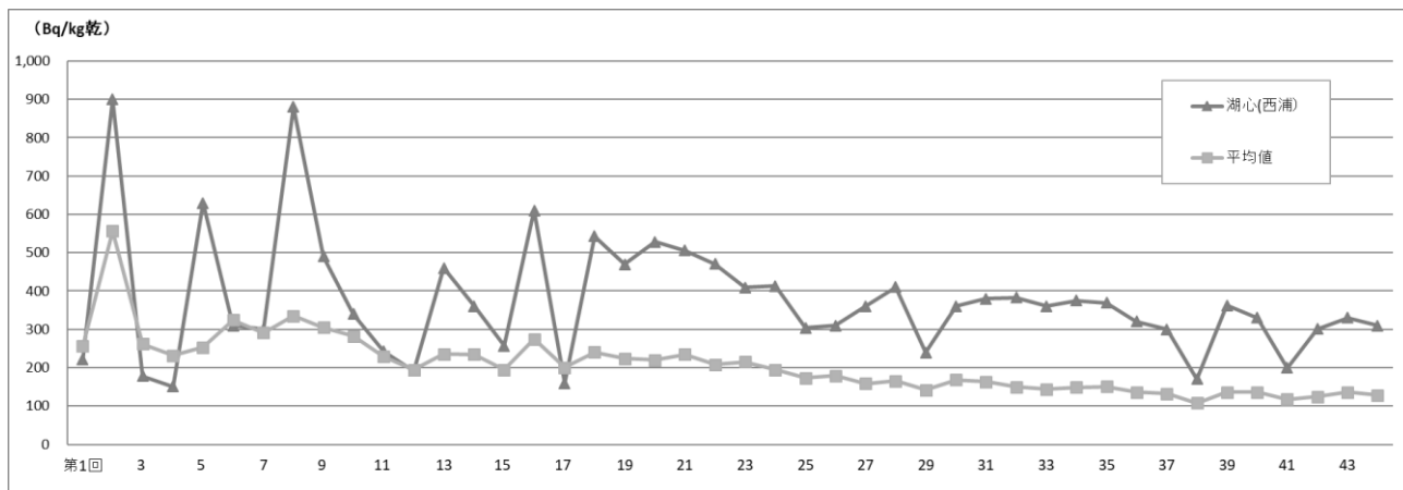
放射性セシウム (セシウム 134+セシウム 137) 濃度が最も高かった湖心 (西浦) の測定値と平均値の推移
